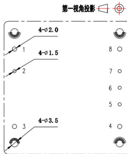
推荐PCB开槽尺寸
