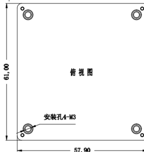
标准型 61*57.9*12.7mm
